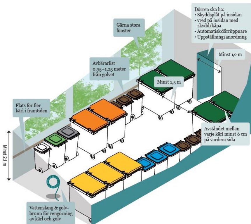
Bild 4 Avfallsutrymme
