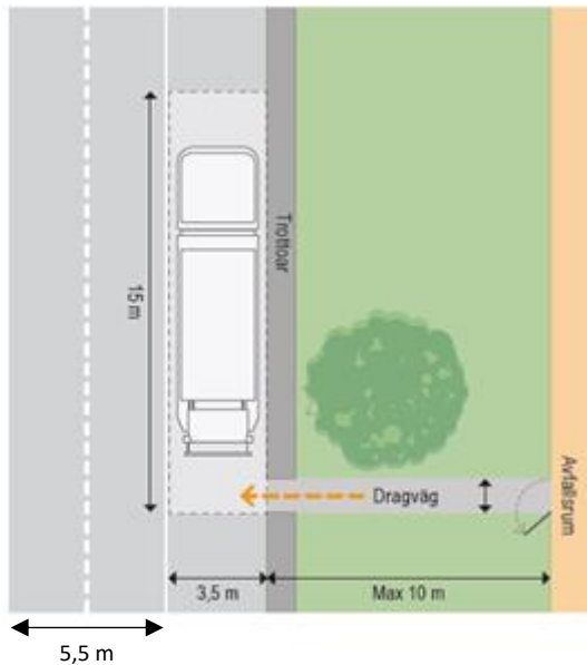
Bild 2 Transportväg
