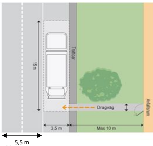
Bild 2 Transportväg
