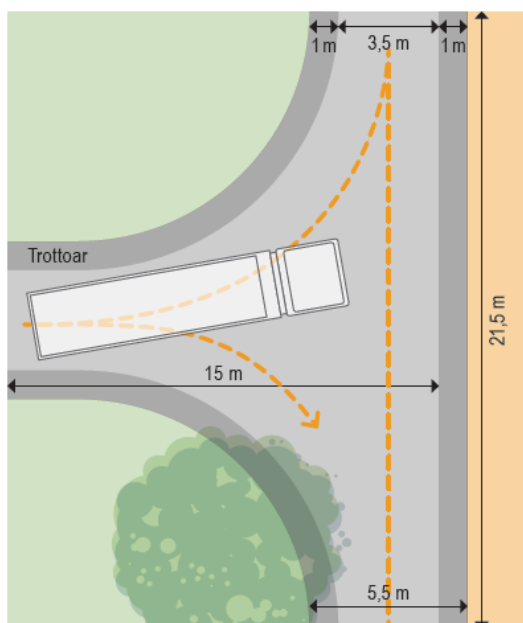
Bild 5 T-korsvändning
