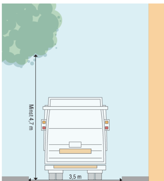
Bild 3 Frihöjd
